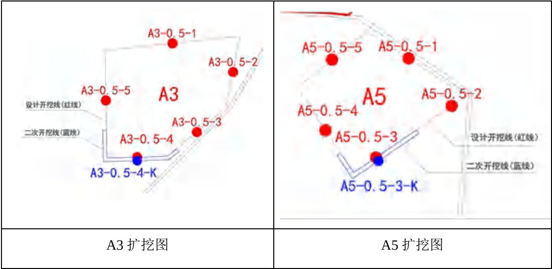
图 3.5-20 第一层（0-1m）设计范围与实际范围对比图
