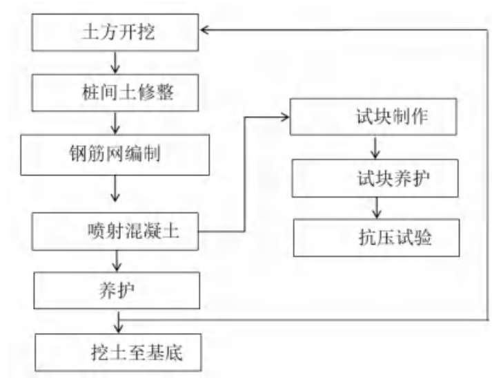
图 3.5-5 施工流程图
