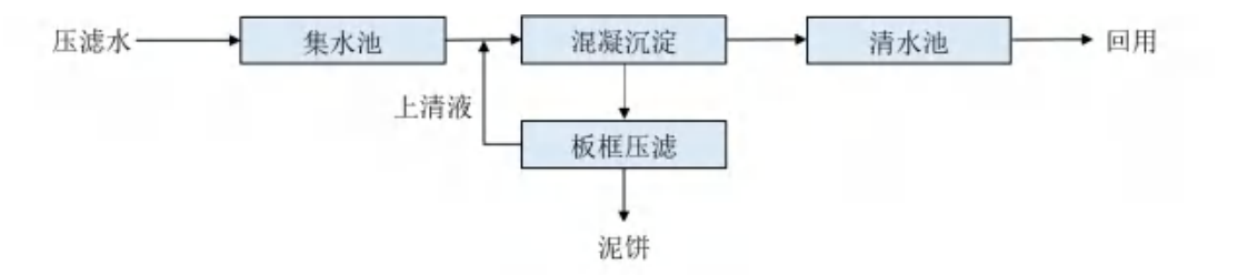
图 3.6-19 废水处理工艺流程图
