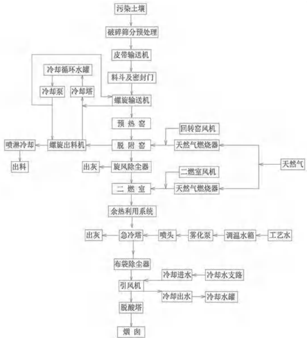
图 2.3-13 热脱附系统工艺流程图
