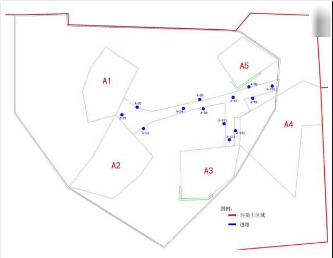
图 3.5-42 第一层施工便道平面图
