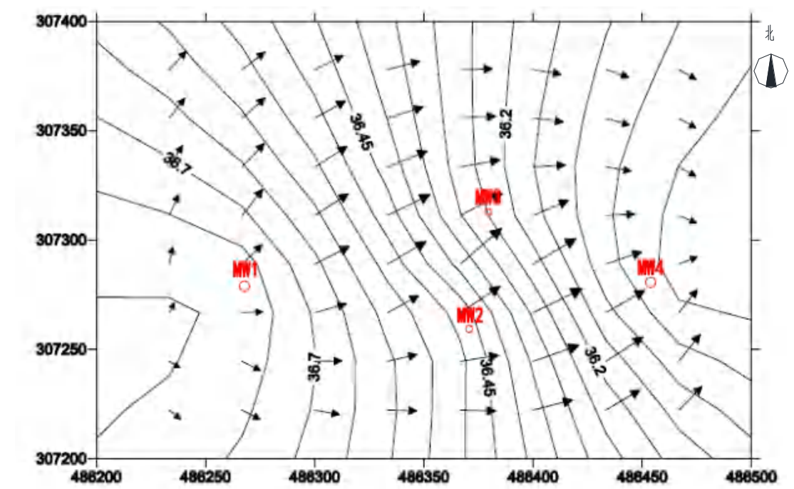
图 2.1-18 地块地下水（潜水）水位标高等值线图
